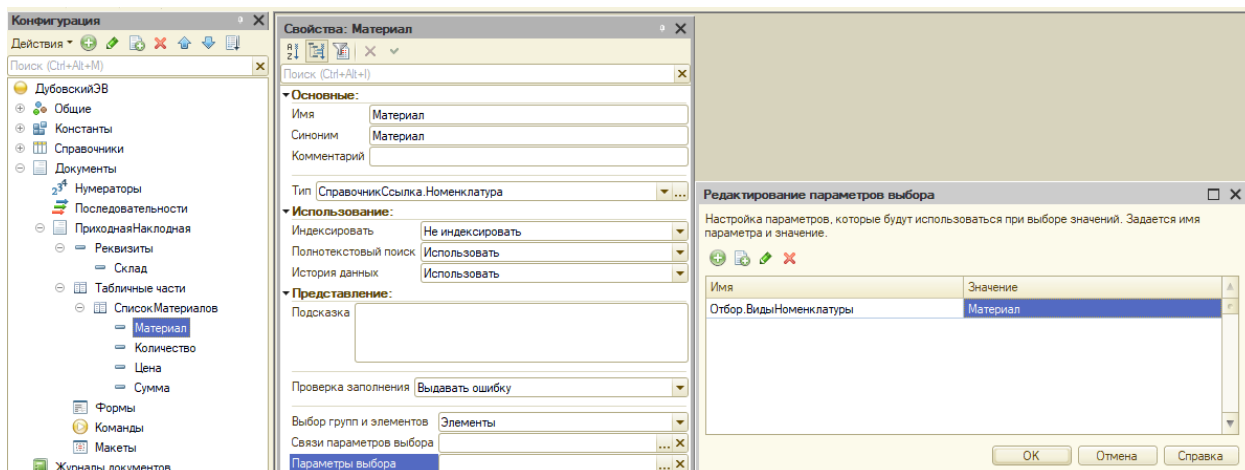
Рисунок 10 – Настройка свойств реквизита “Материал” в “СписокМатериалов”
