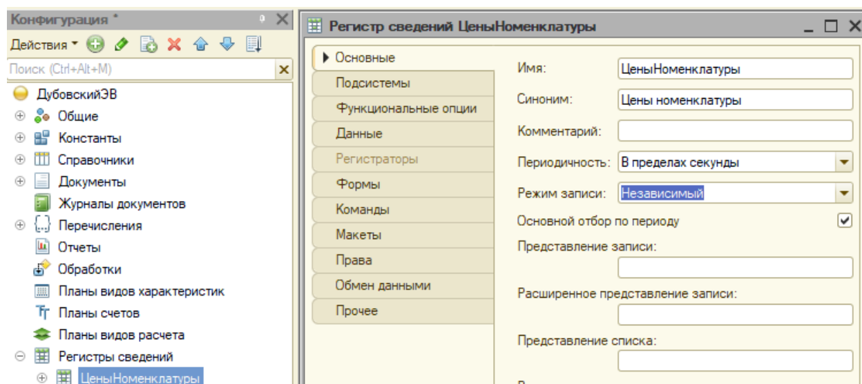
Рисунок 28 – Создание регистра сведений “ЦеныНоменклатуры”
