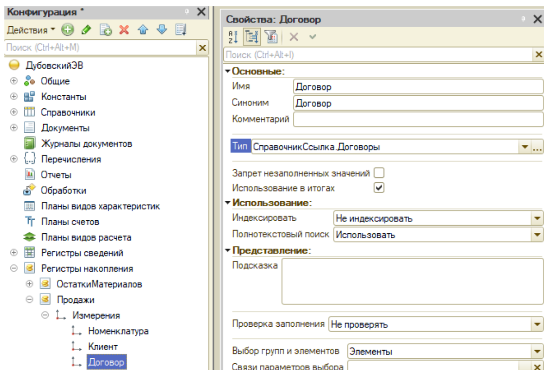
Рисунок 45 – Создание измерения “Договор”
