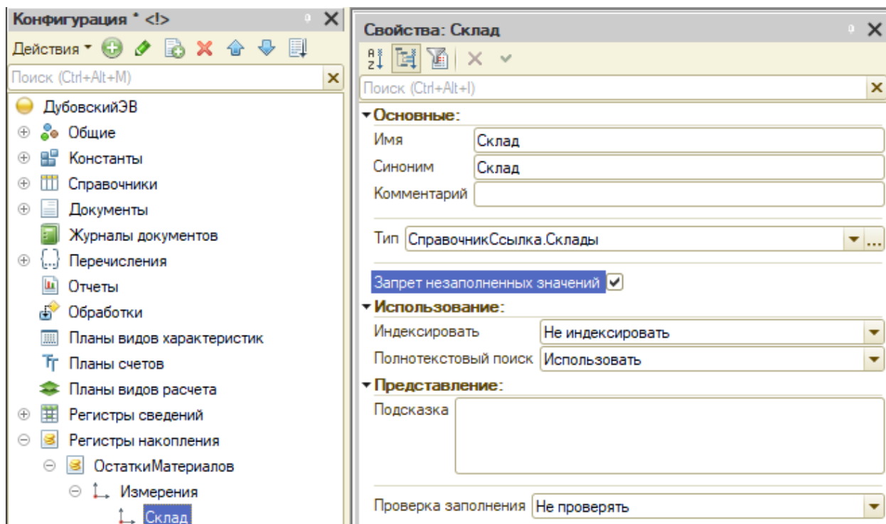
Рисунок 36 – Создание измерения “Склад”
