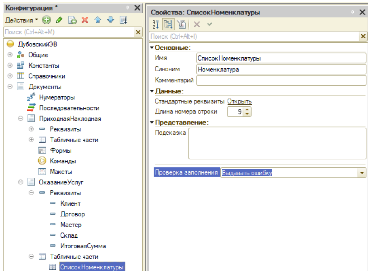
Рисунок 19 – Создание “СписокНоменклатуры” в табличной части
