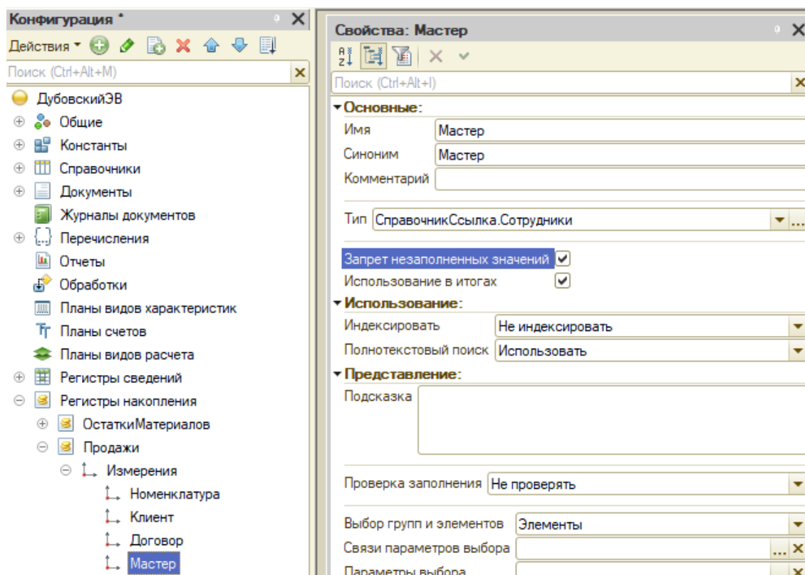
Рисунок 46 – Создание измерения “Мастер”
