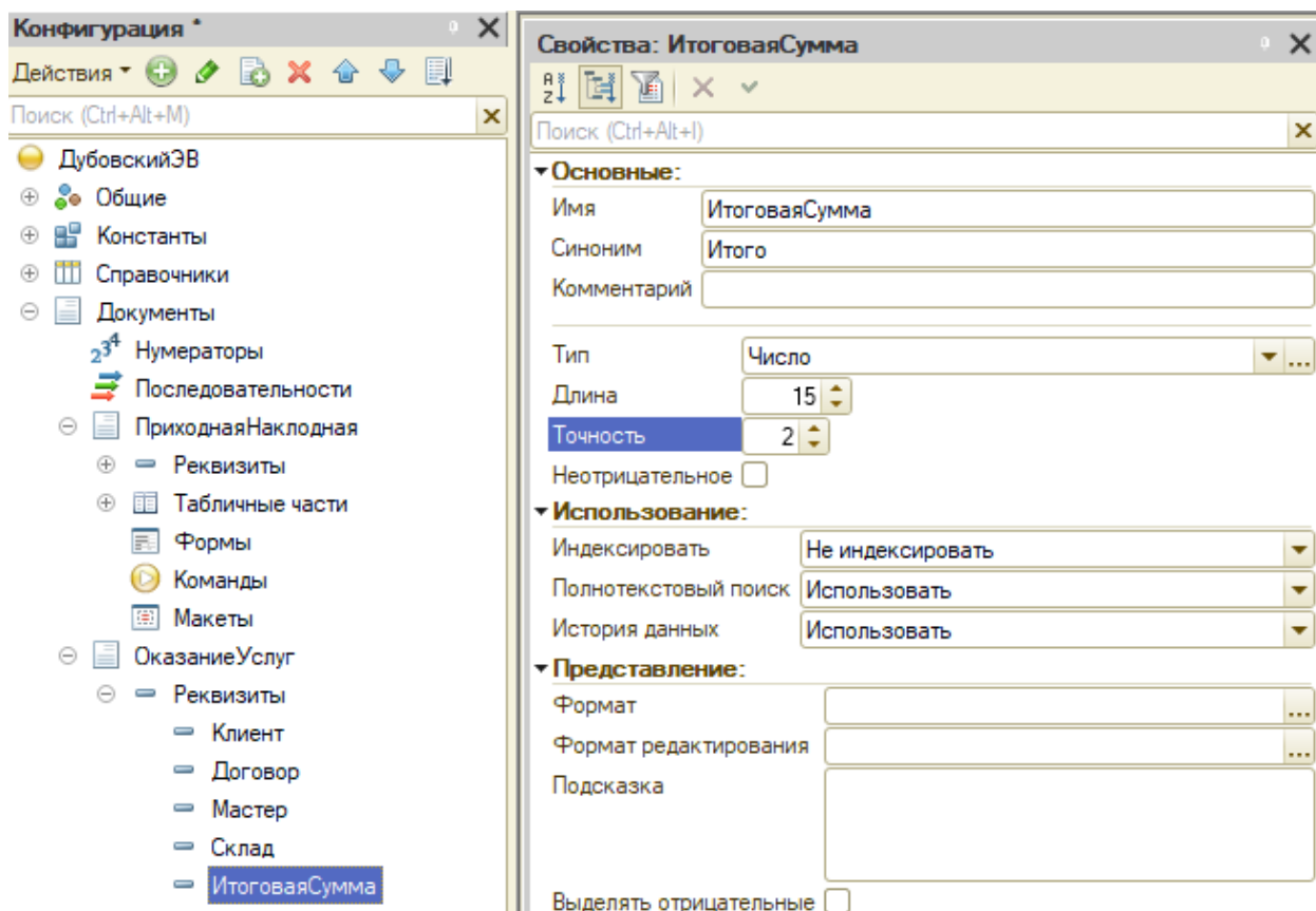
Рисунок 18 – Создание реквизита “ИтоговаяСумма”
