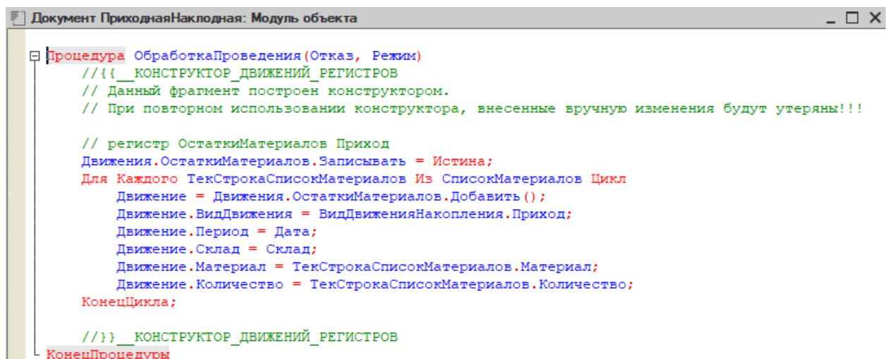
Рисунок 49 – Использование конструктора движений для “ПриходнаяНакладная”
