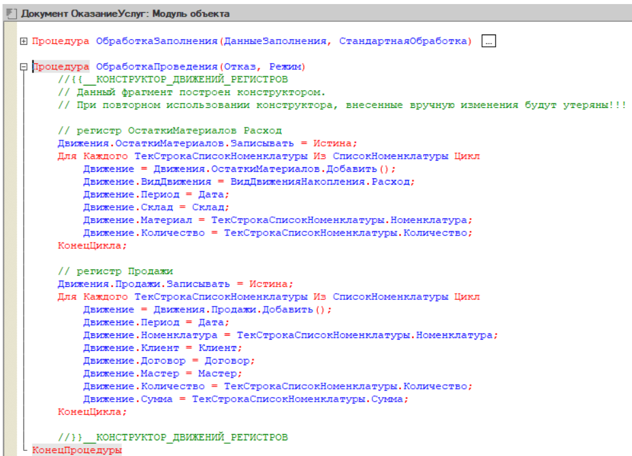
Рисунок 52 – Документ “ОказаниеУслуг” модуль объекта
