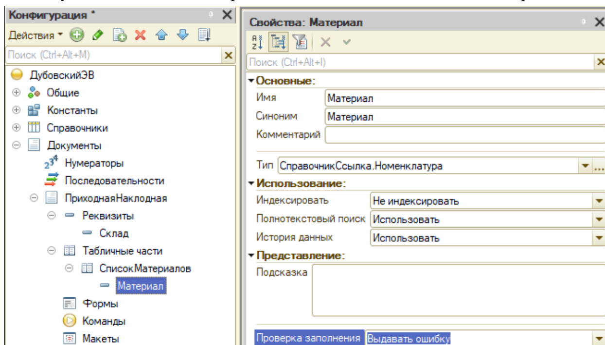
Рисунок 6 – Настройка реквизитов “Материал” в “СписокМатериалов”
