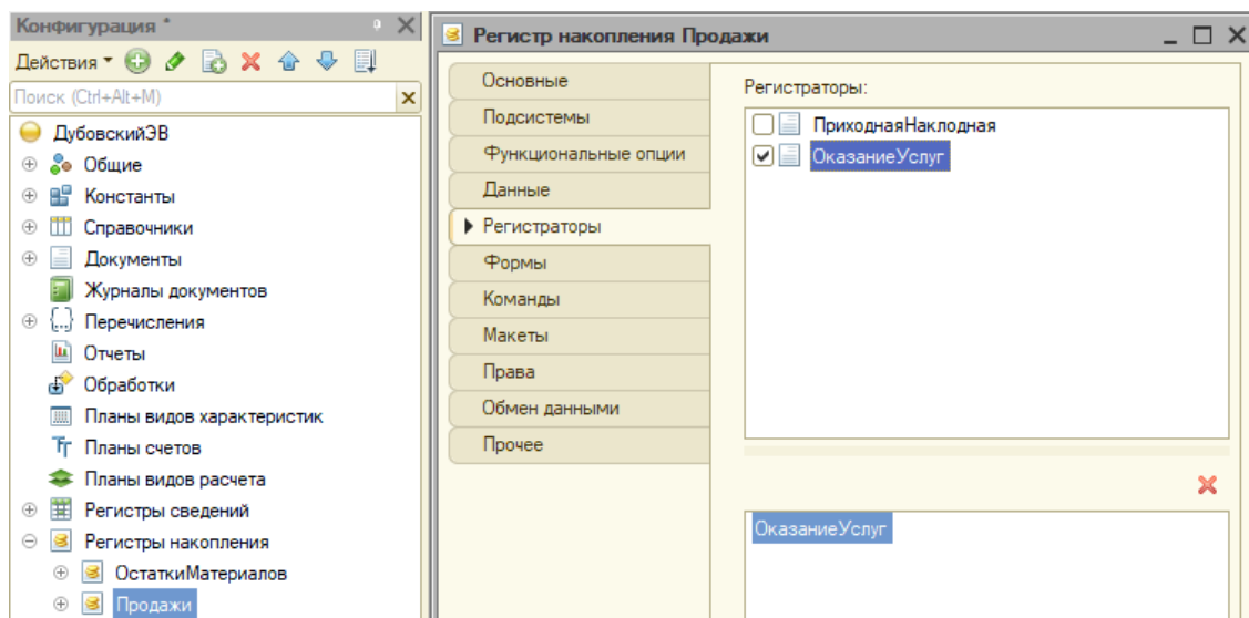
Рисунок 40 – Создание регистра накопления “Продажи”
