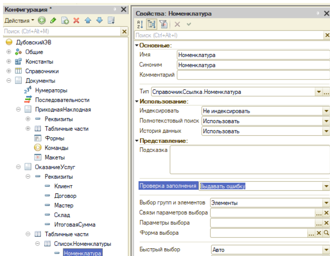
Рисунок 21 – Создание реквизита “Номенклатура”
