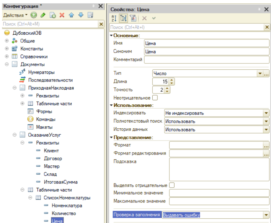
Рисунок 23 – Создание реквизита “Цена”
