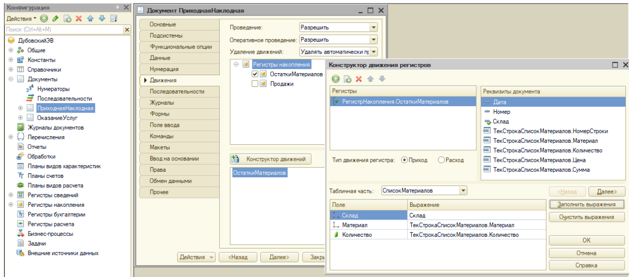
Рисунок 49 – Использование конструктора движений для “ПриходнаяНакладная”
