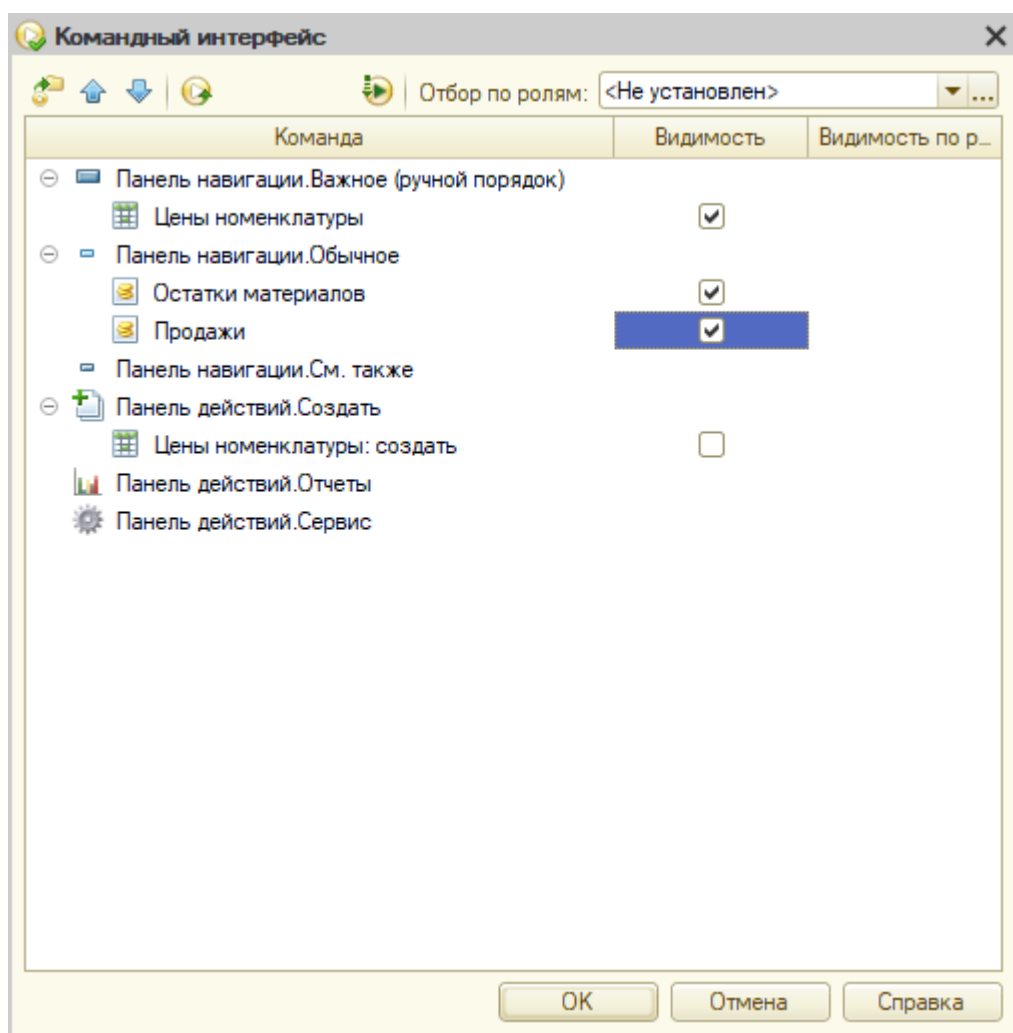
Рисунок 55 – Настройка командного интерфейса “Регистры”
