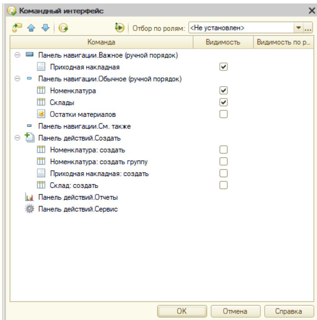
Рисунок 53 – Настройка командного интерфейса “УчетМатериалов”
