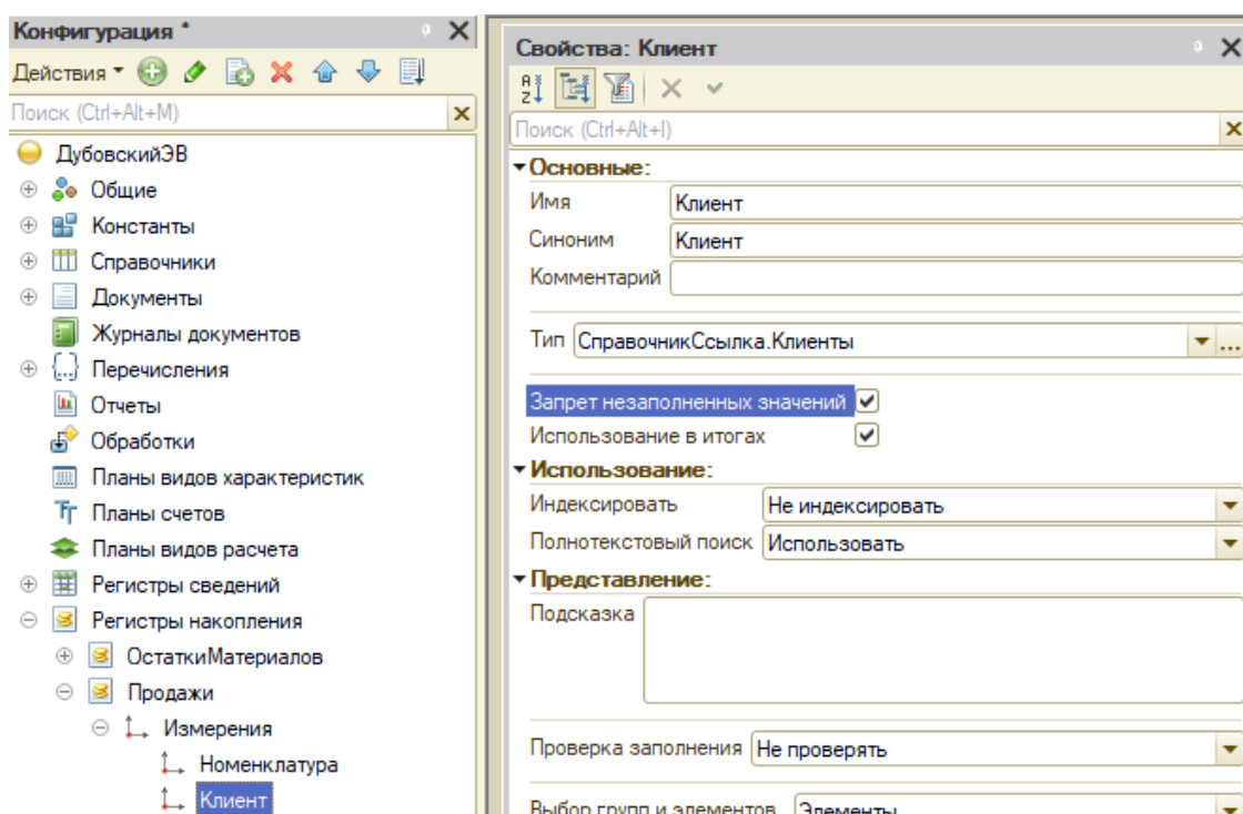
Рисунок 44 – Создание измерения “Клиенты”
