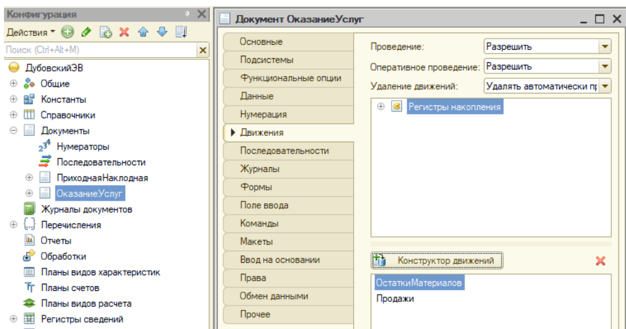
Рисунок 51 – Использование конструктора движений для “ОказаниеУслуг”
