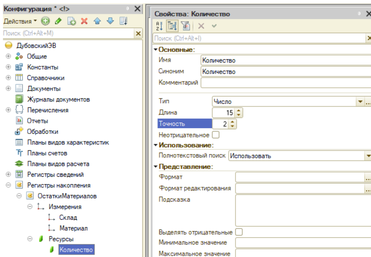
Рисунок 38 – Создание ресурса “Количество”
