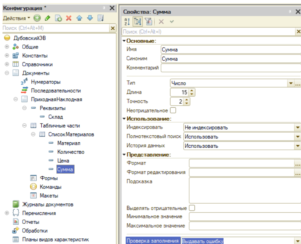
Рисунок 9 – Настройка реквизитов “Сумма” в “СписокМатериалов”
