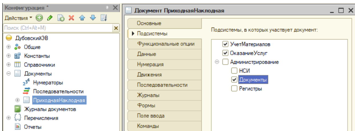
Рисунок 2 – Настройка документа “ПриходнаяНакладная”
