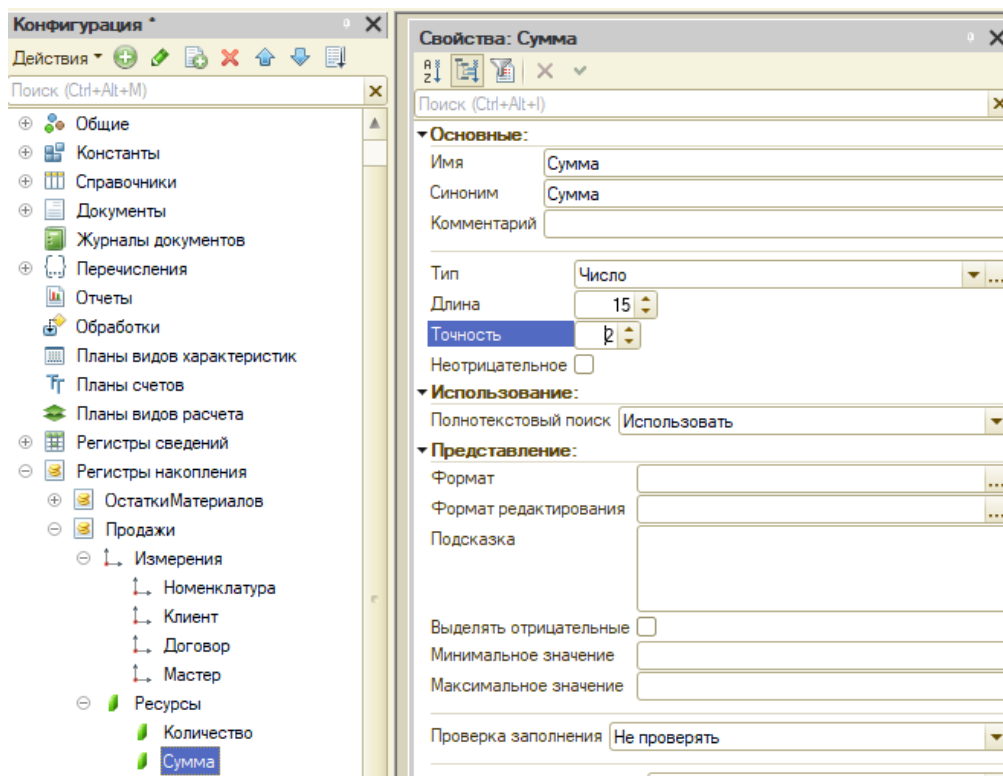
Рисунок 48 – Создание ресурса “Сумма”
