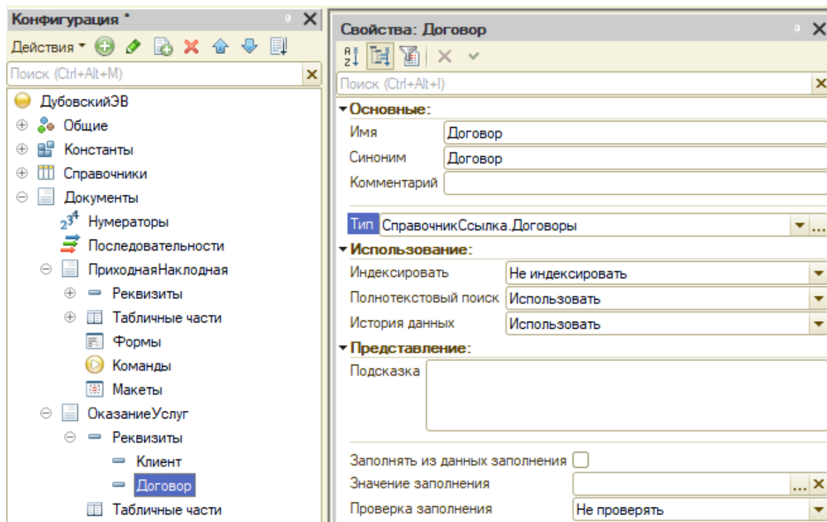
Рисунок 15 – Создание реквизита “Договор”
