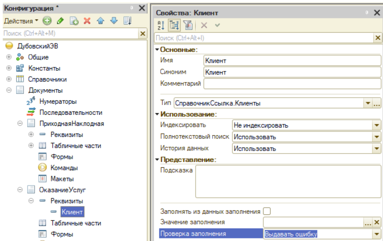
Рисунок 14 – Создание реквизита “Клиент”
