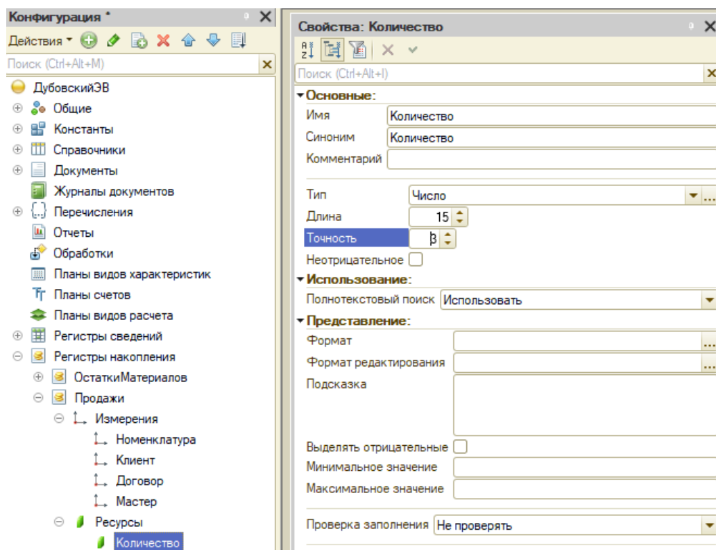
Рисунок 47 – Создание ресурса “Количество”
