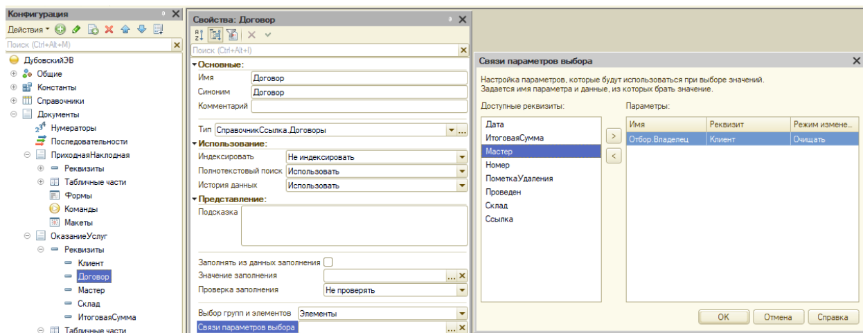
Рисунок 25 – Настройка свойства “Договора”
