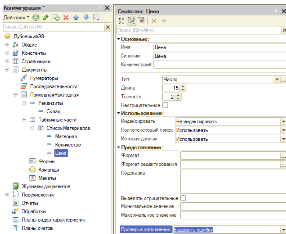
Рисунок 8 – Настройка реквизитов “Цена” в “СписокМатериалов”
