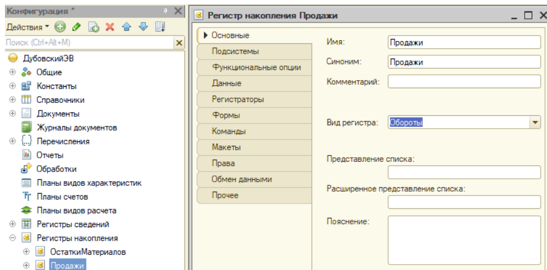
Рисунок 39 – Создание регистра накопления “Продажи”
