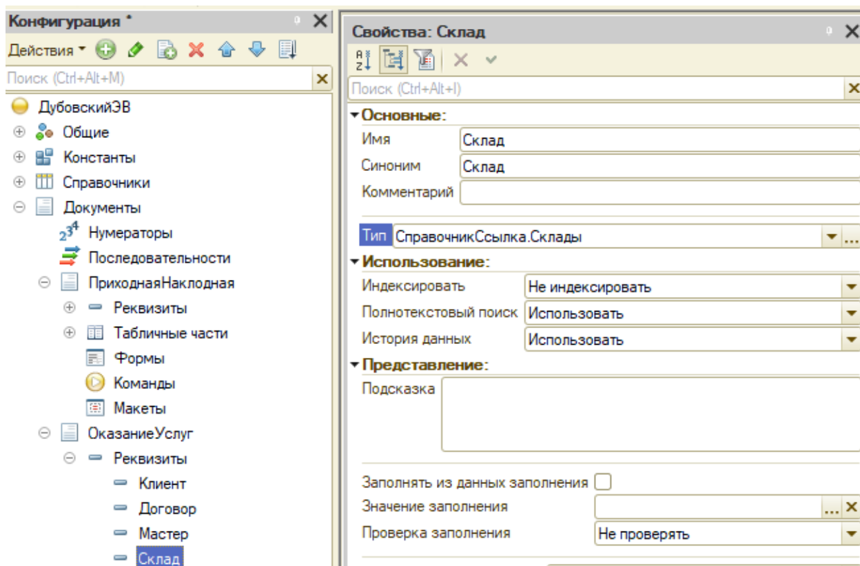
Рисунок 17 – Создание реквизита “Склад”
