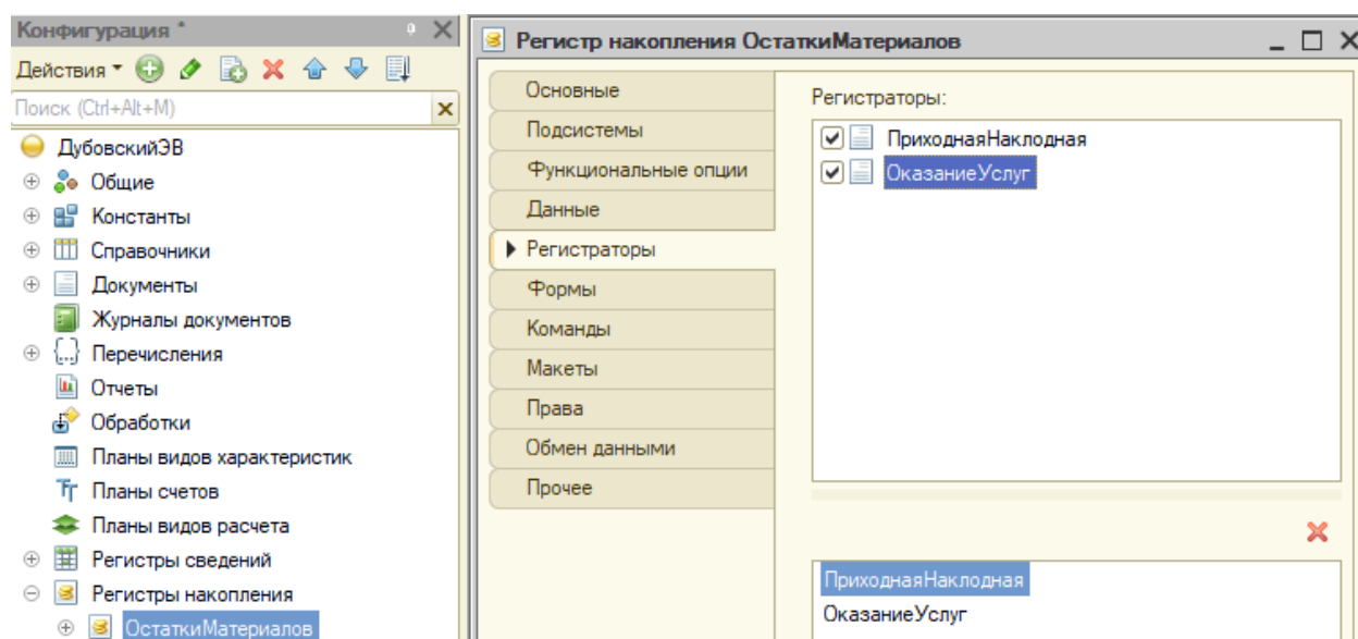
Рисунок 33 – Настройка регистра накопления “ОстаткиМатериалов”
