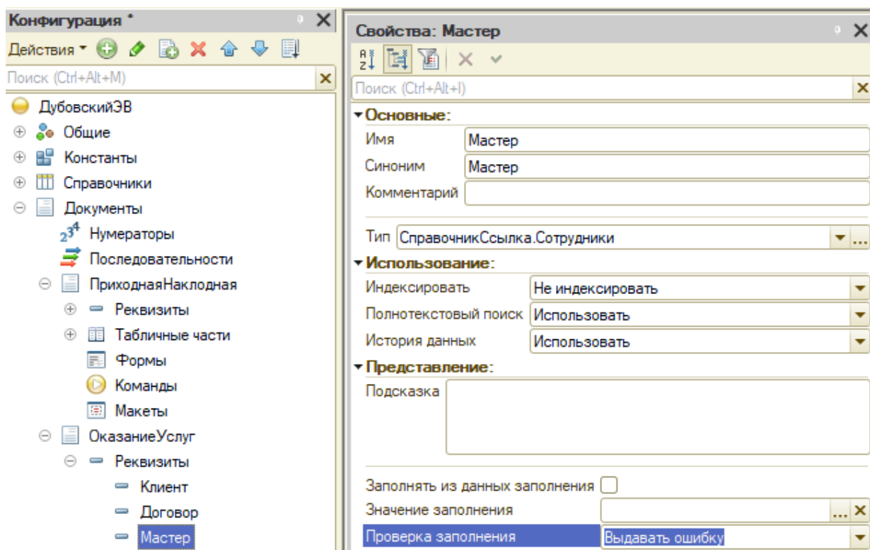
Рисунок 16 – Создание реквизита “Мастер”
