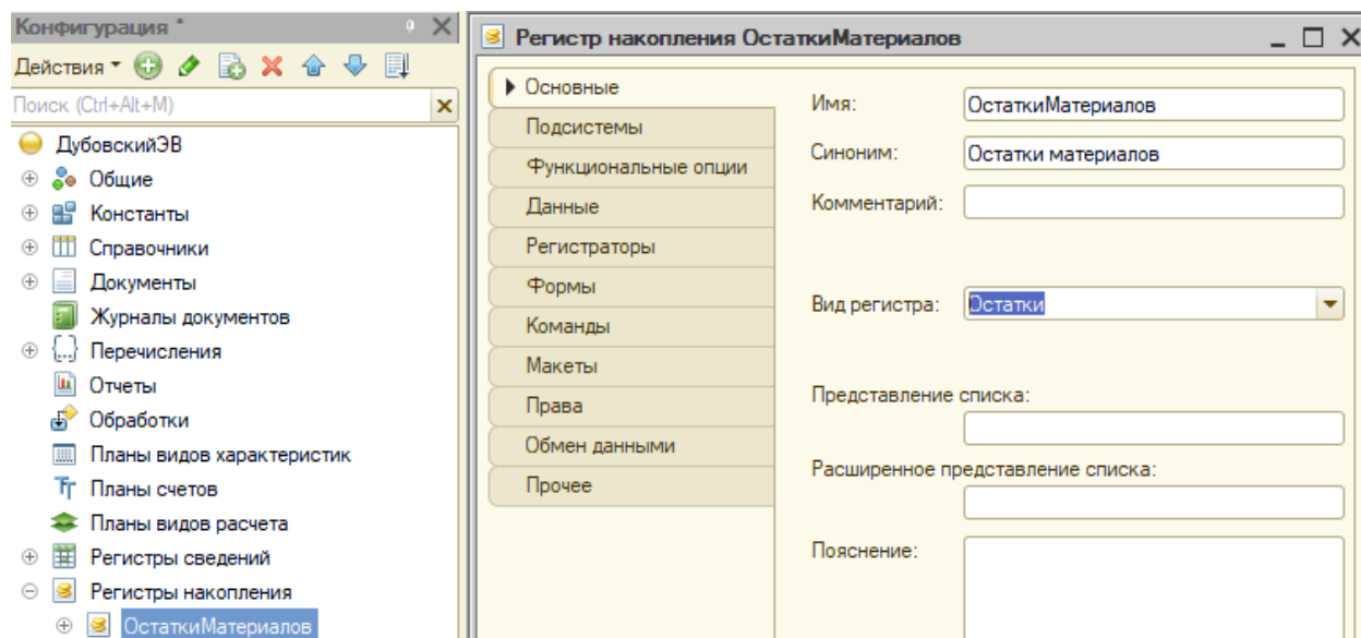
Рисунок 32 – Настройка регистра накопления “ОстаткиМатериалов”
