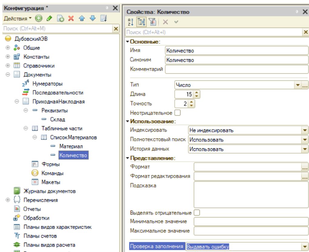
Рисунок 7 – Настройка реквизитов “Количество” в “СписокМатериалов”
